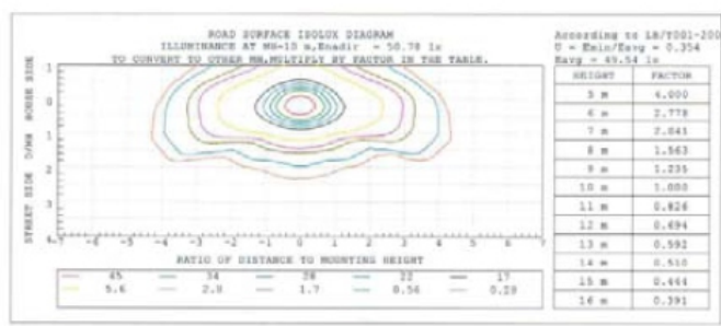
แผนภาพแสดงแสงสว่างที่พื้นบริเวณ
