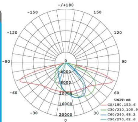
แผนภาพแสดงเส้นความส่องสว่างเพาบนมิวออน
