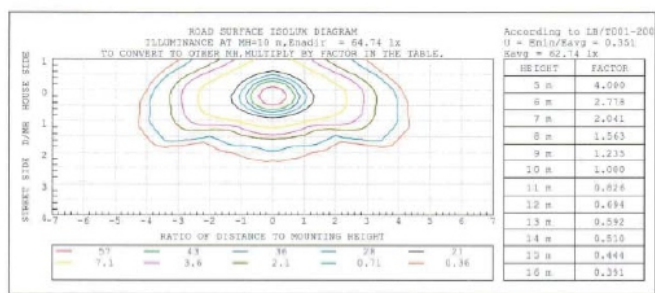
แผนภาพแสดงเส้นความส่องสว่างเท่ากันบริเวณ
